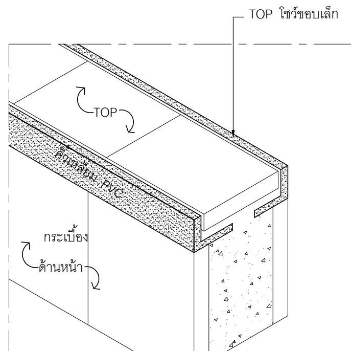
DETAIL (D4) ธรณีกันสวนเปียก/สวนแห้ง
