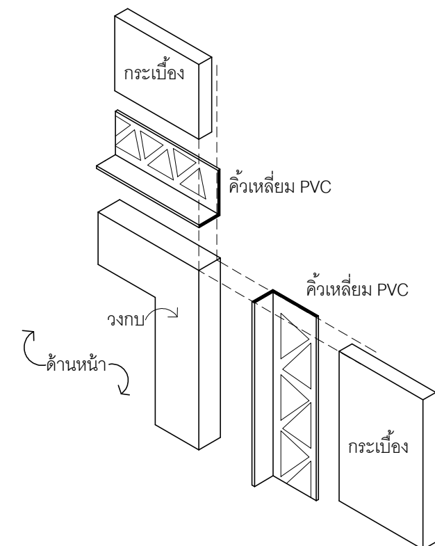
DETAIL (D6) คิวรอบวงกบ
