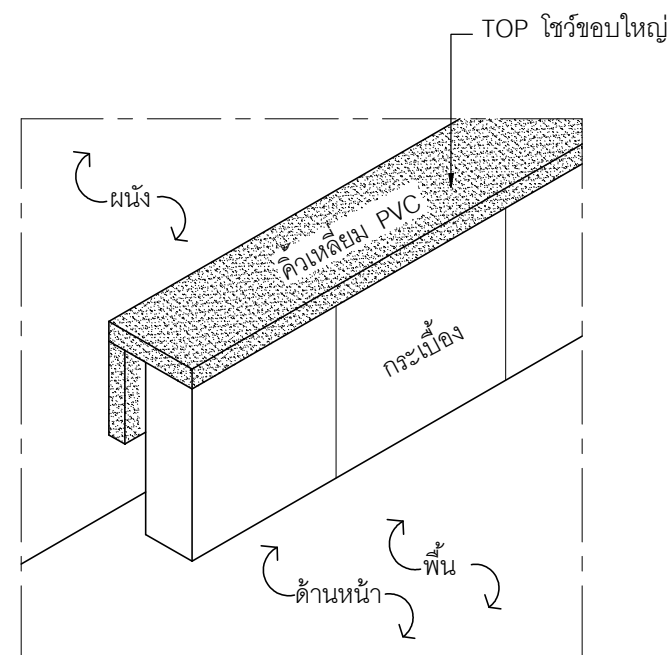
DETAIL (D2) บัวกันเปื้อน
