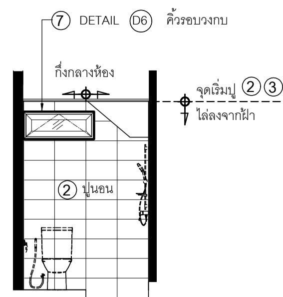
รูปตัด (3) 1 : 50
