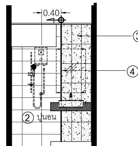
รูปตัด (4) 1 : 50
