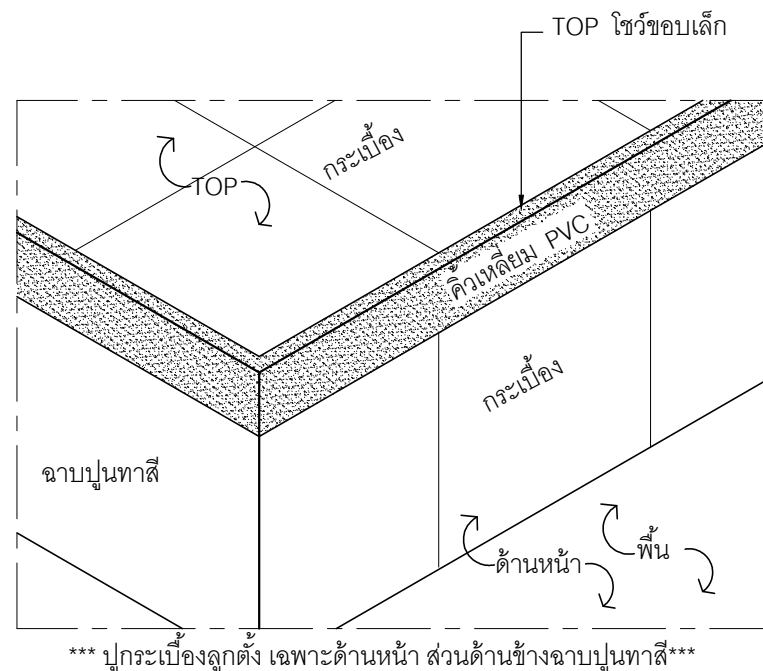
DETAIL (D1) STEP บั๊นได
