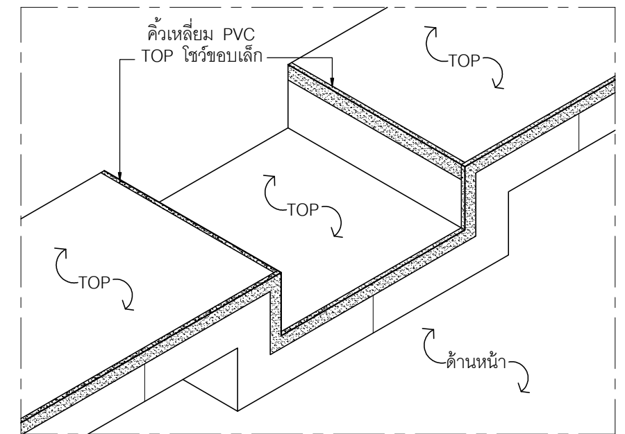
DETAIL (D3) TOP ครีวไทย
