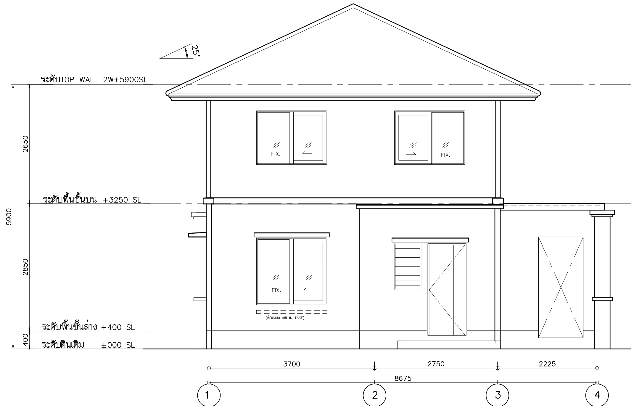
รูปด้าน 3 1:50
