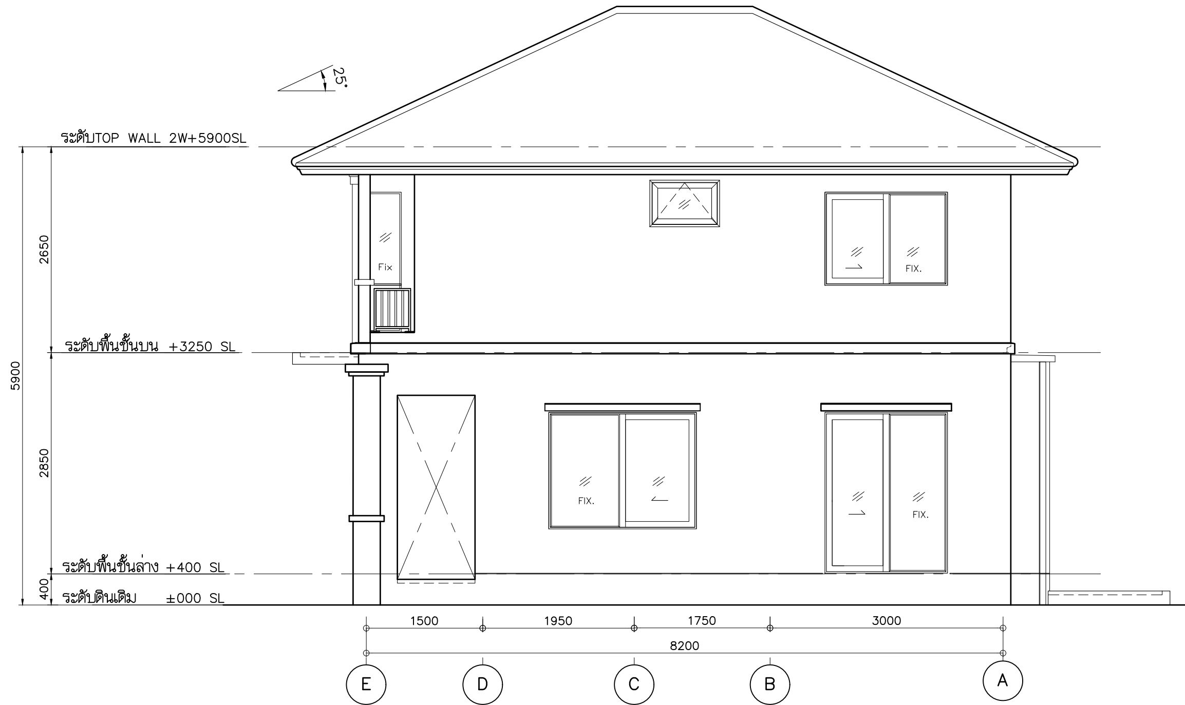
รูปด้าน 2 1:50
